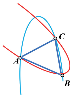
1-chizma. Parabola ga ichki chizilgan uchburchak
